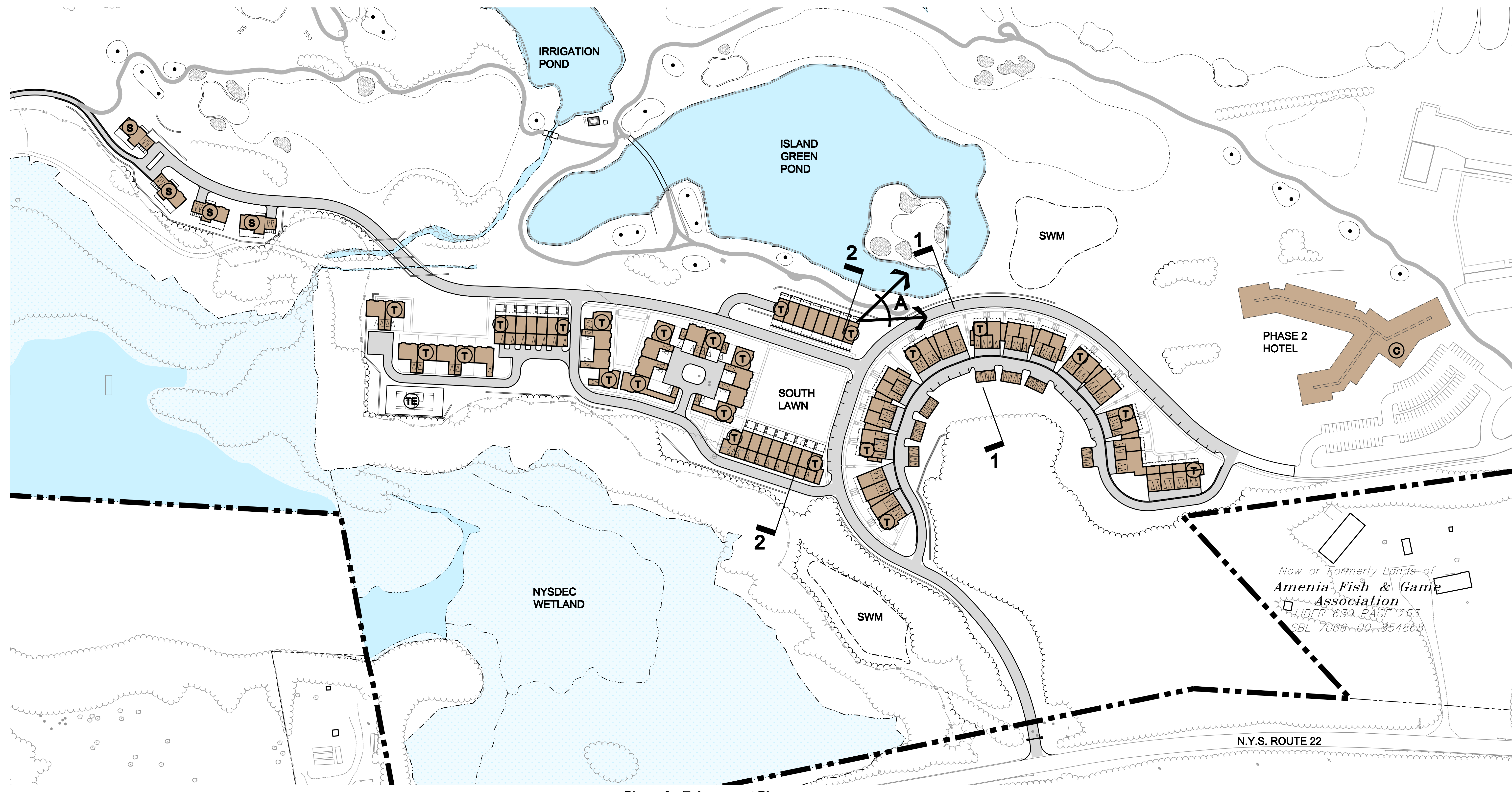
Phase 2 - Enlargement Plan
